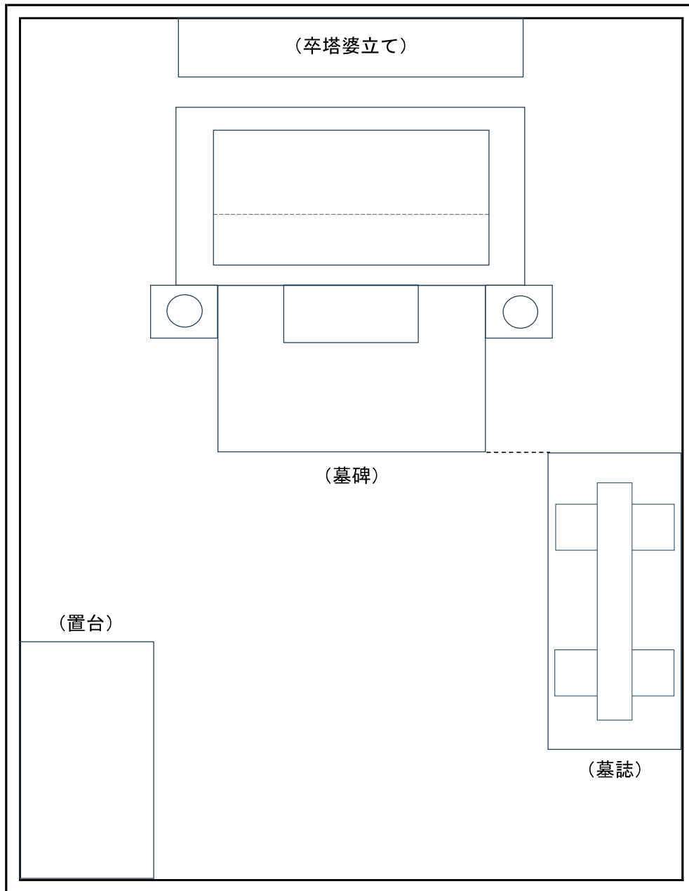
配置（平面図）
