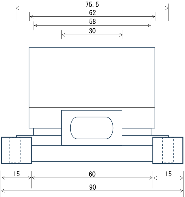
(正面図)
