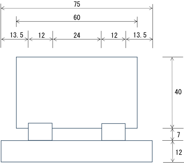
(正面図)
