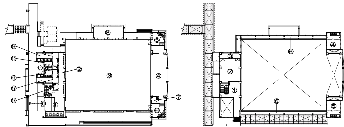
1階平面図
